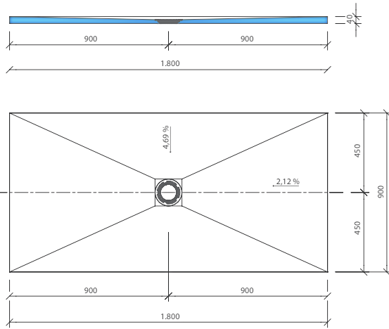
Primo shower element
