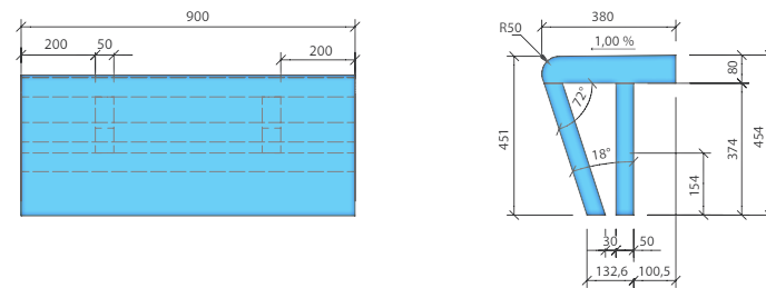
Sanoasa bench 3, rounded edge
